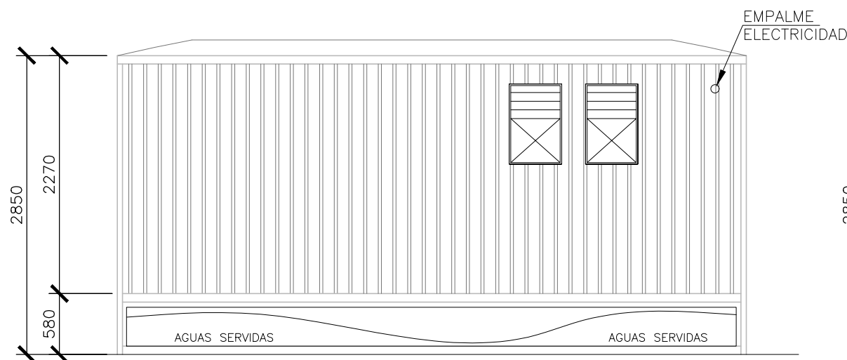
ELEVACIÓN NORTE
