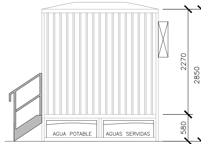
ELEVACIÓN ESTE
