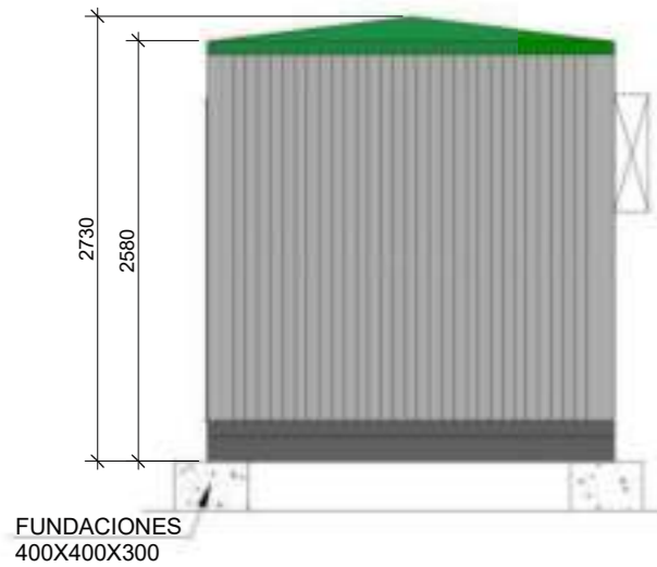
ELEVACION ESTE
