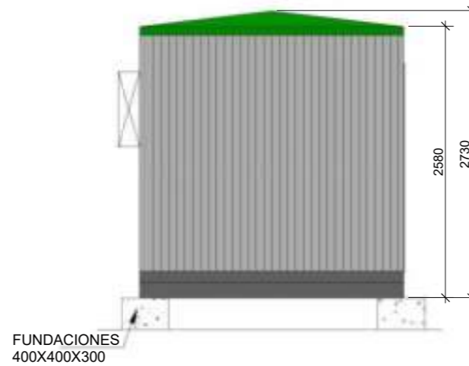
ELEVACION OESTE
