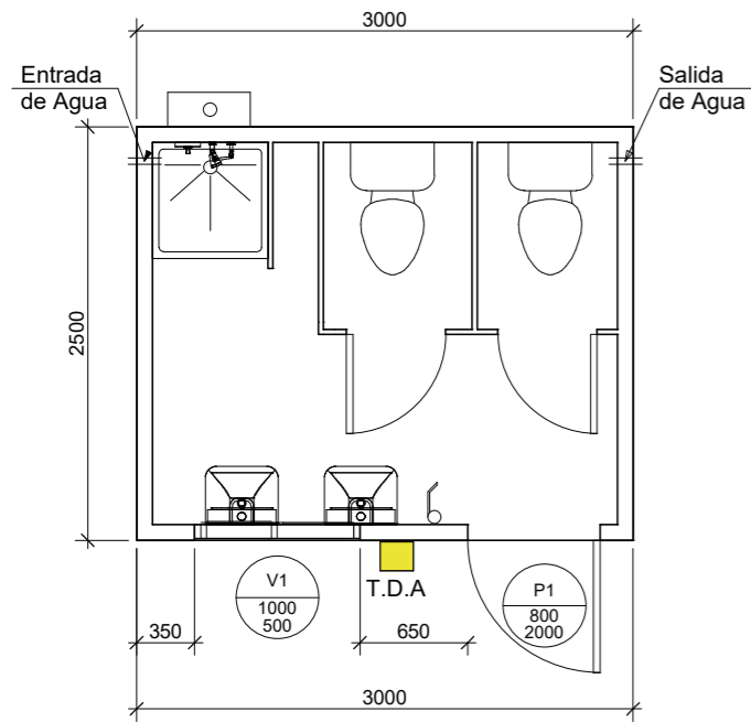
PLANTA
