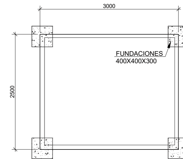
PLANTA FUNDACIONES
