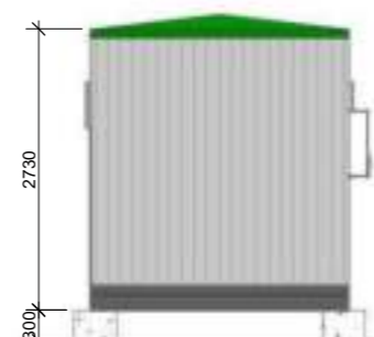
ELEVACION ESTE
